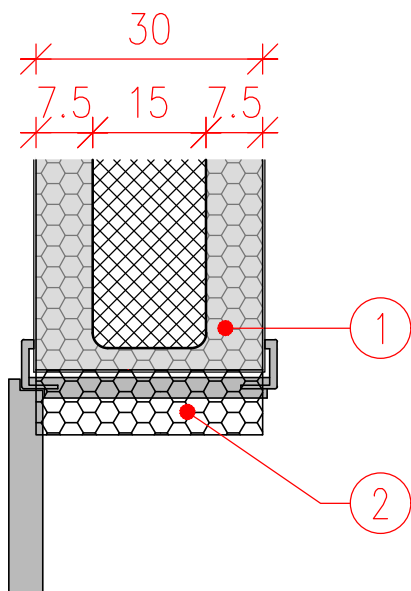
PREREZ PREKLADE – REZANJE
