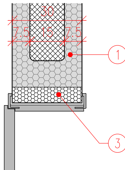
PREREZ PREKLADE – LEPLJENJE
